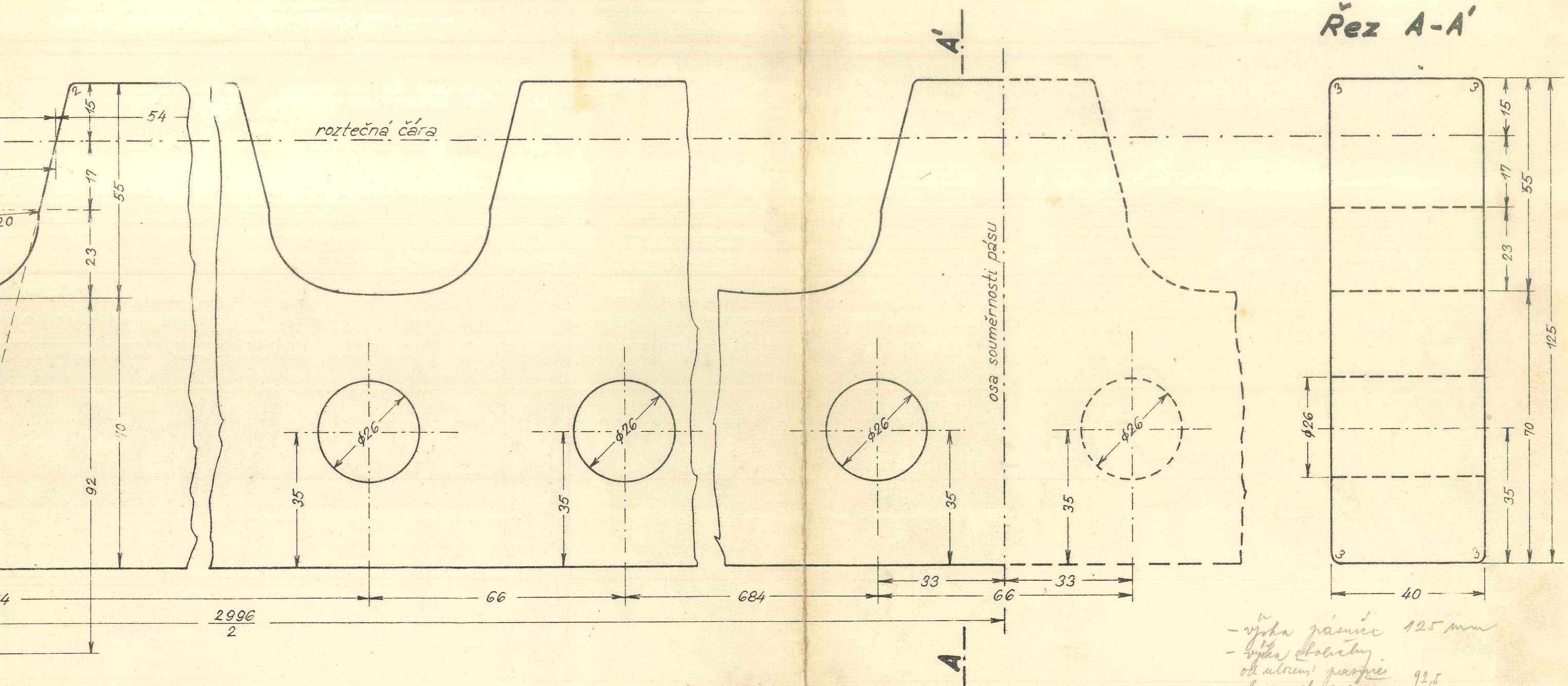
Obr. 1. Detail ozubnicového pásu 1:1
